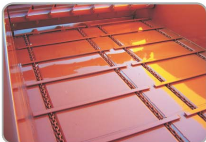
Esteira Rolante: Movimenta o material para descarga dianteira ou traseira.
