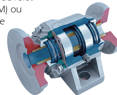
Rolamentos de Rolos Cônicos e Retentores Duo-Cone .
