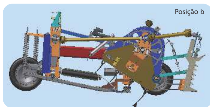
Posição do molinete que levanta as plantas tombadas para frente.
