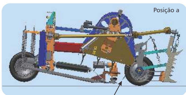
Posição normal do molinete
